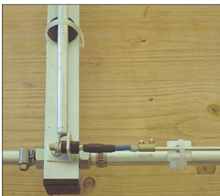
Bild 6: Isoliert angebrachte Telefonbuchse am Boom mit angeschlossenen 6-mm-Phasenleitungsrohr
