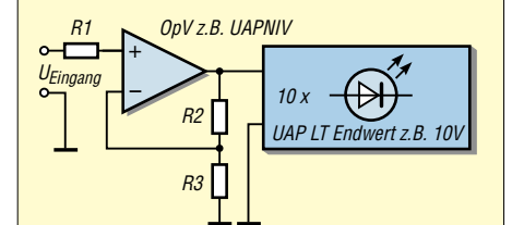
Bild 67: Messspannung im mV-Bereich
