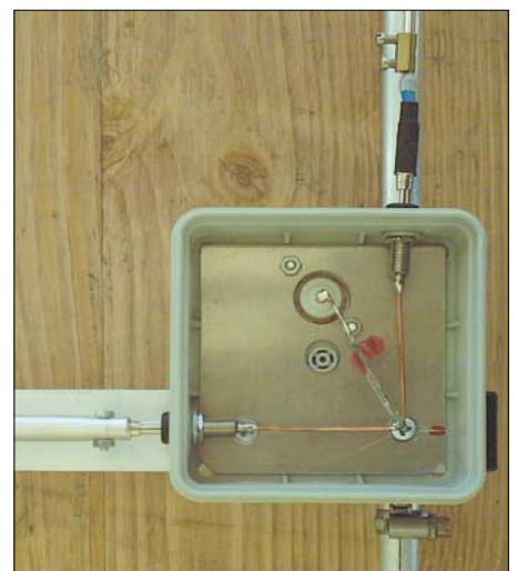
Bild 4: Innenansicht der Anschlussdose mit PL- und Bananenbuchsen
