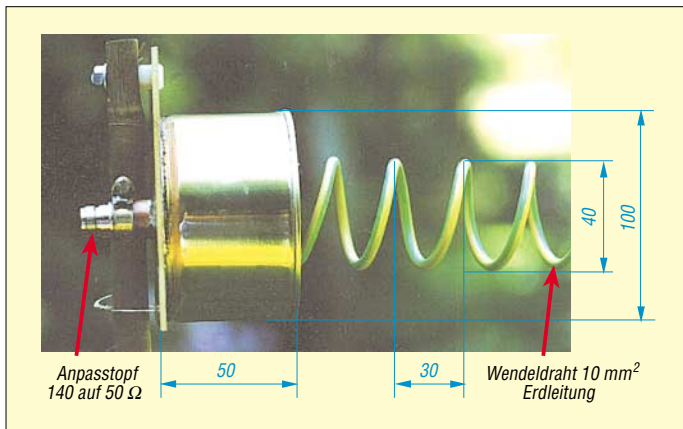
Bild 9: Helix-Feeder im Topf, geeignet für Offsetspiegel mit f/D = 0,7
