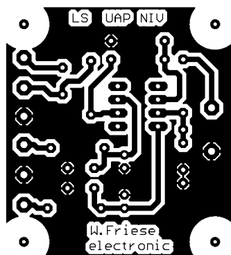
Bild 80: Leiterseite der Platine UAP NIV im Maßstab 1:1
