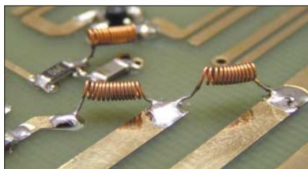
Bild 2: Die auf den Schaft eines Bohrers gewickelten Viertelwellendrosseln sind mit einem kleinen Abstand zur Platine einzulöten.
