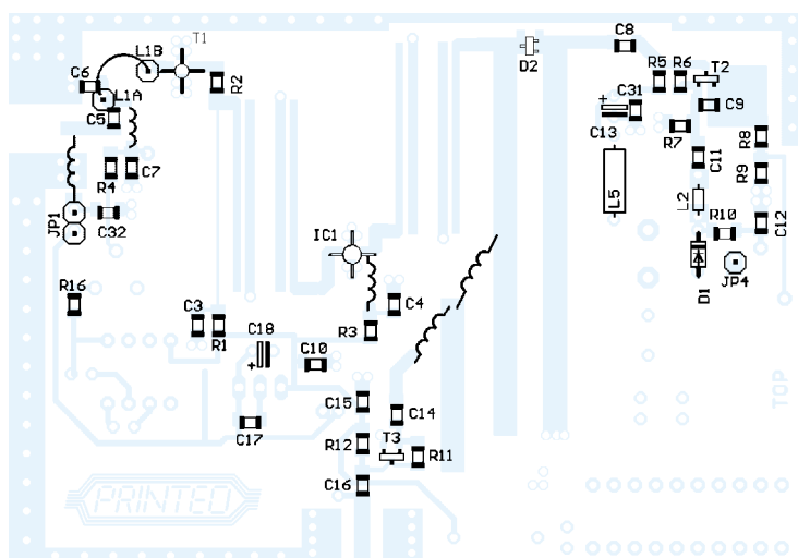
Bild 7: Bestückung auf der Platinenoberseite mit dem Analogteil; die verwendeten SMD-Bauteile lassen sich auf Grund des vorhandenen Platzes gut auflöten.
