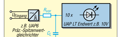
Bild 69: Schaltung zur Anzeige des Spitzenwertes der Eingangsspannung
