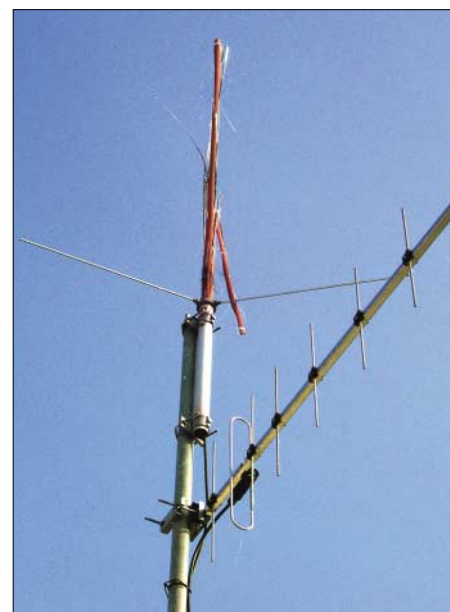
Die X7000 (5 m) des QTC-Autors nach dem Blitzschlag (nur noch knapp 1 m lang). Foto: DL9HQH
