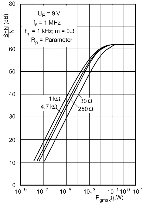
Bild 3: Signal-Rausch-Abstand als Funktion der Generatoreistung am Eingang
