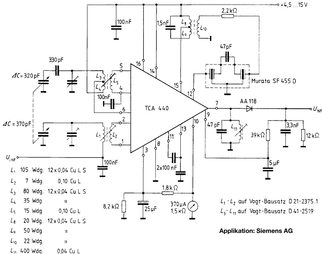
Bild 5: Anwendungsbeispiel für den Empfang der Mittelwelle mit Vorstufenregelung, die aus der ZF abgeleitet wird
