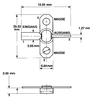
230 mil BeO
