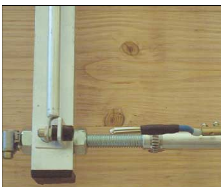
Bild 7: Steckbarer Übergang der Phasenleitung vom Boom zum Reflektor
