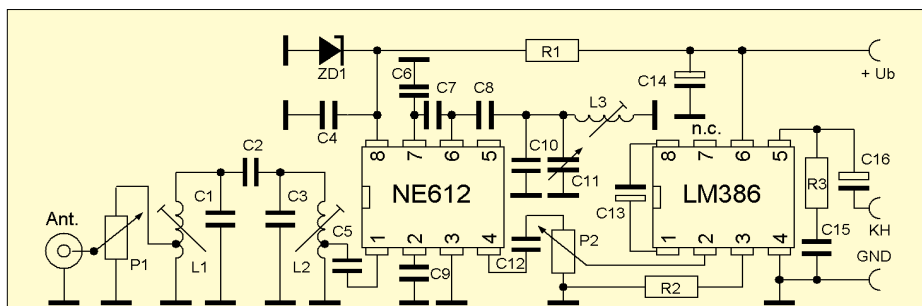
Bild 4: Das übersichtliche Schaltbild eines mit sPlan 5.0 gezeichneten Direktmischempfangers verdeutlicht den Vorteil gegenüber einer Handskizze.
