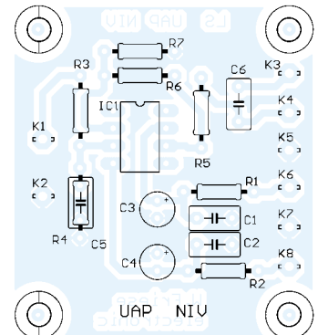
Bild 81: Bestückungsplan der einseitigen Platine UAP NIV
